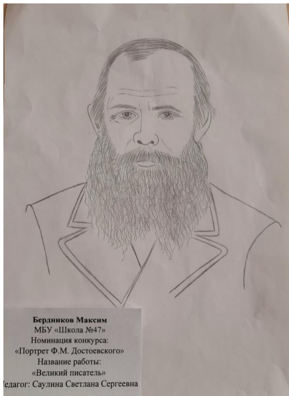
Портрет Ф.М. Достоевского. Бердников Максим, 2 класс МБУ «Школа № 47»
